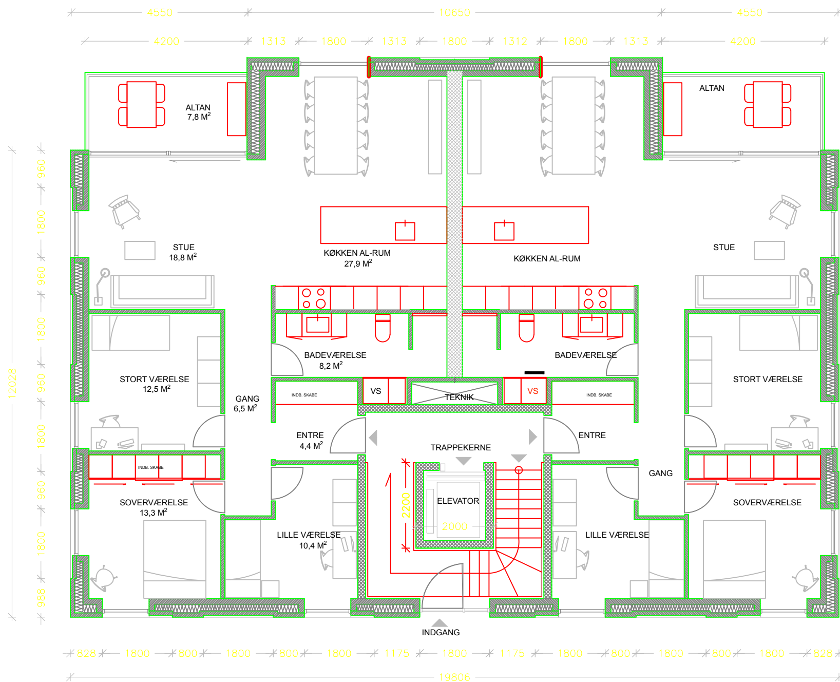
PLANTEGNING 1:100 STUEPLAN - 3 ETAGE
